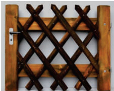
Scherenzauntor mit Kastenschloss DIN links
